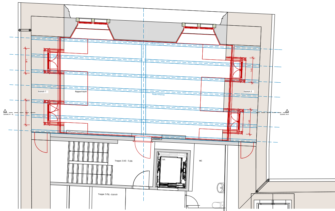
Grundriss Rapportraum 3.OG
