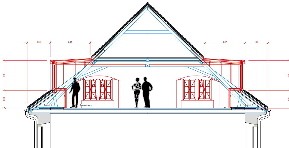
Schnitt A-A Rapportraum 3.OG
